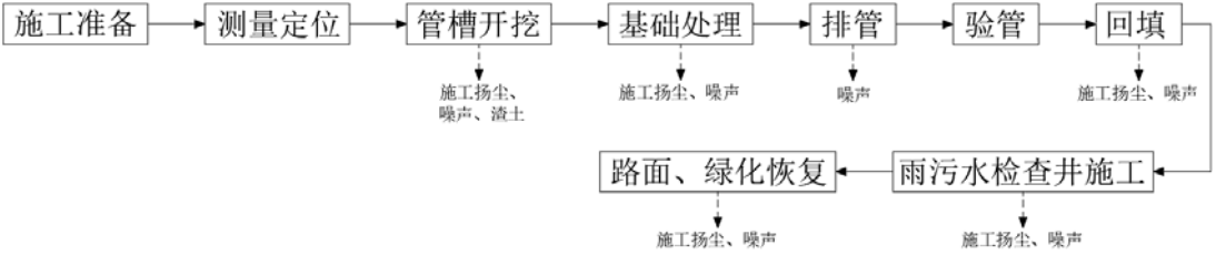
图 2-5 雨污管道施工工艺流程图
