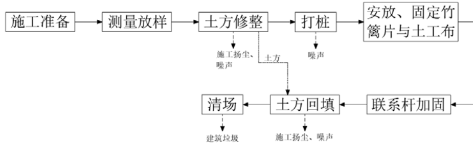
图 2-4 河道护岸施工工艺流程图
