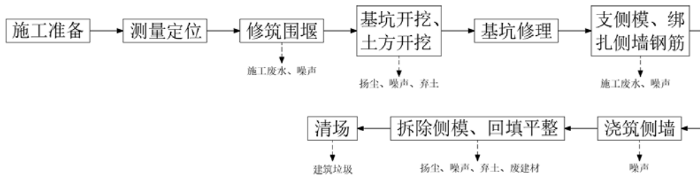
图 2-1 河道开挖、新建挡墙工艺流程图
