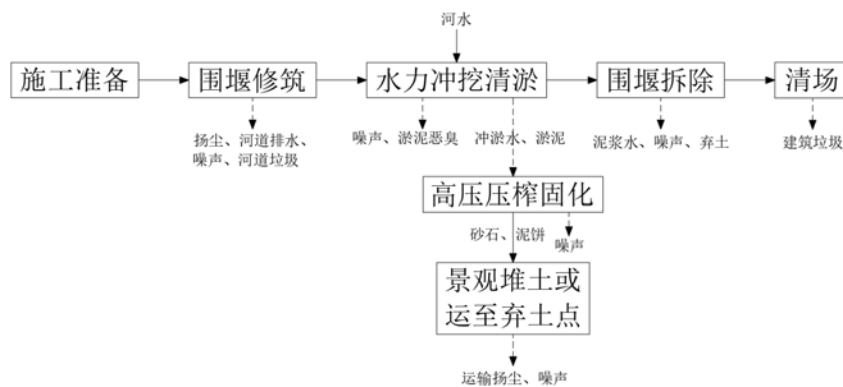
图 2-2 河道清淤工艺流程图
