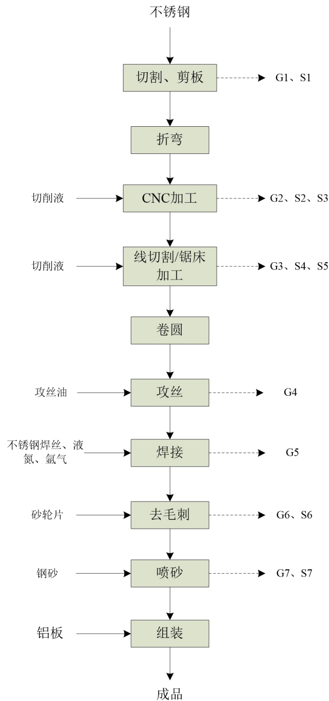
图 2-2 成型器、机架及电气箱、安装支架生产线工艺及产污环节图 工艺流程说明：
