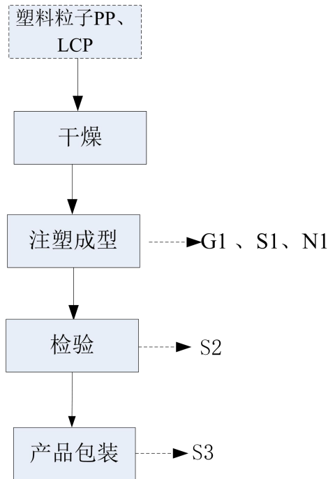
图 2-2 接插件、连接器生产工艺流程图
