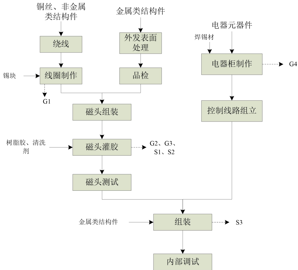
图 2-1 检针机（半成品）生产工艺及产污环节图
