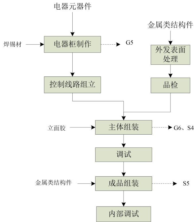
图 2-2 缝制设备（粘合机、射频读码装置等）生产工艺及产污环节图 工艺流程说明：
