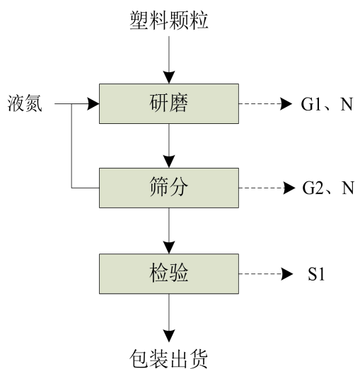
图 2-2 3D 新型材料的生产工艺及产污环节图
