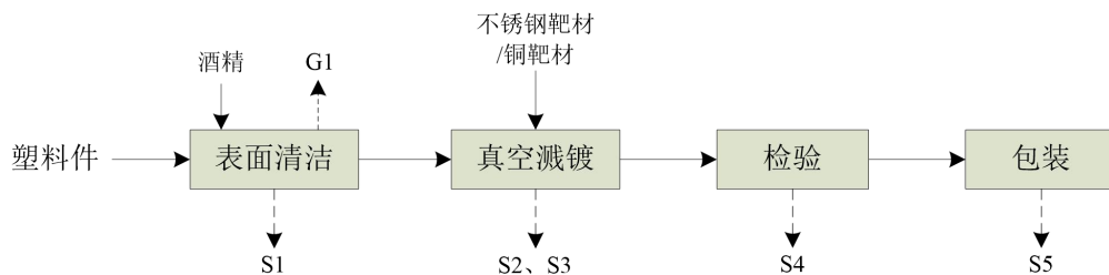
图 2-2 电子元器件生产线工艺及产污环节图
