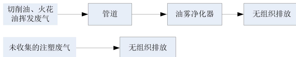
图4-2 本项目无组织废气收集、治理走向图本项目
