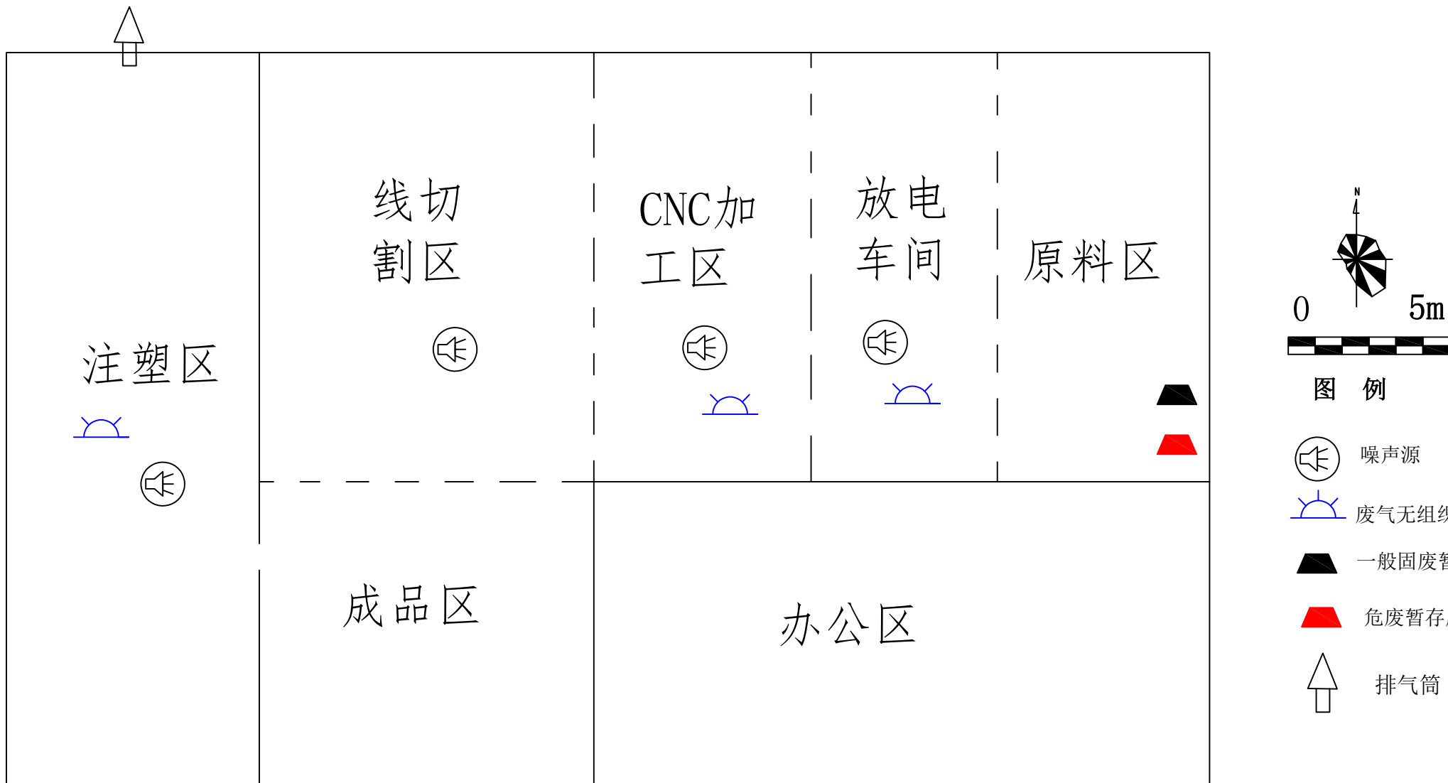
附图4 车间平面布局图
