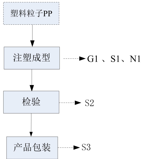
图 2-2 塑料量杯生产工艺流程图
