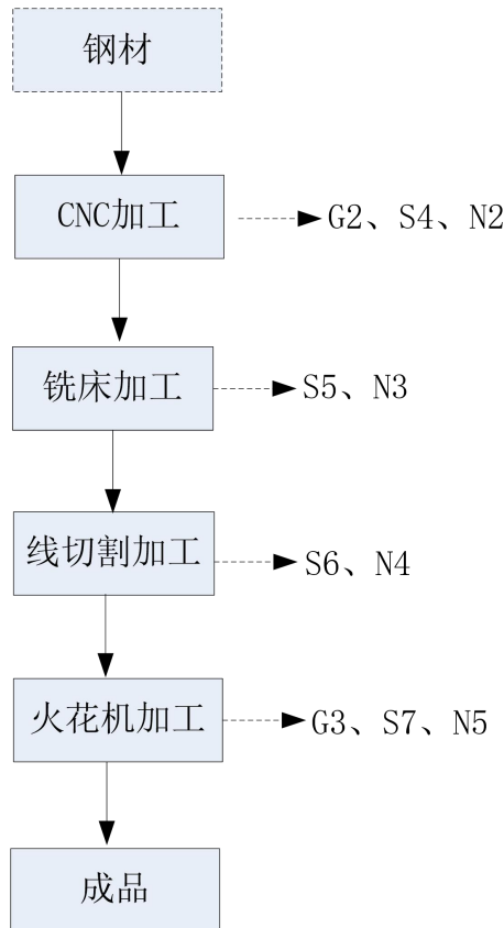
图 2-3 模具生产工艺流程图
