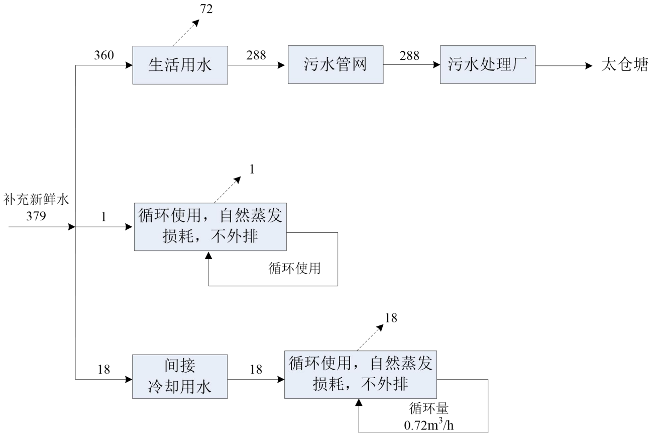
图 2-1 建设项目水平衡图 (单位: t/a)
