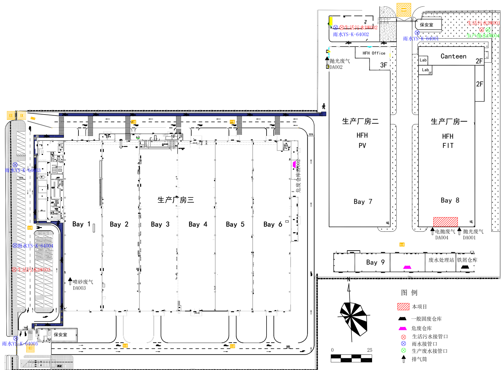
附图4 车间平面图
